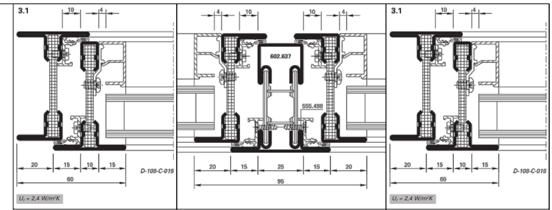
A-A
